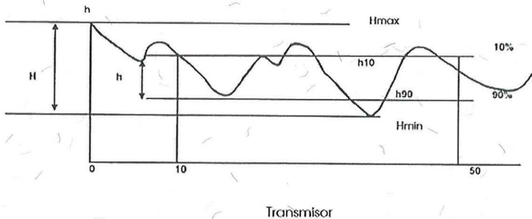
Figura 7. Gráfica de Irregularidad del terreno
