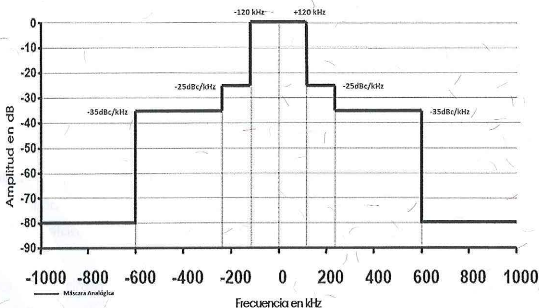
Figura 2. Máscara del espectro de Emisión de una señal de F.M.
