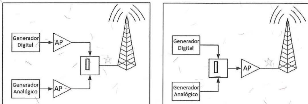
Figura 4. Ejemplos simplificados de sistemas FM híbridos de línea común. Se indica el punto en el que se tomará la muestra de la señal.
