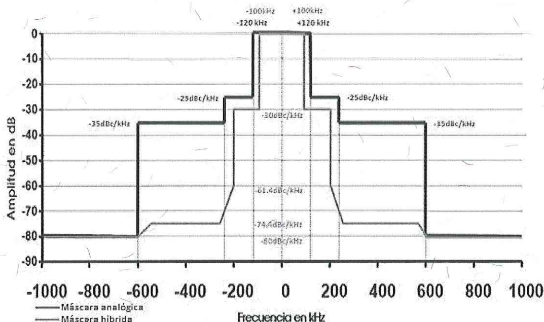
Figura 3. Máscara del espectro de Emisión de una señal F.M. híbrida.
