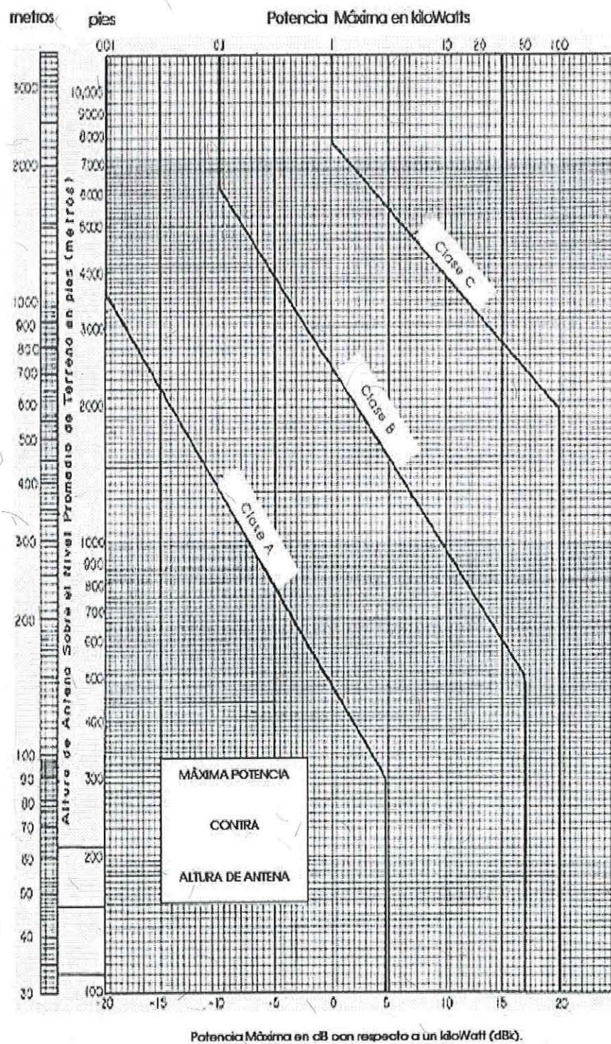
Figura 6. Gráfica de Altura contra Potencia.
