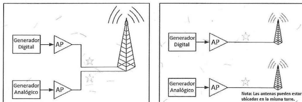
Figura 5. Ejemplos simplificados de sistemas FM híbridos de líneas separadas. Se indica el punto en el que se tomará la muestra de la señal.
