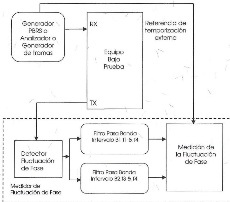
Figura 7. Diagrama para la medición de la fluctuación de fase pico a pico en el puerto de salida
