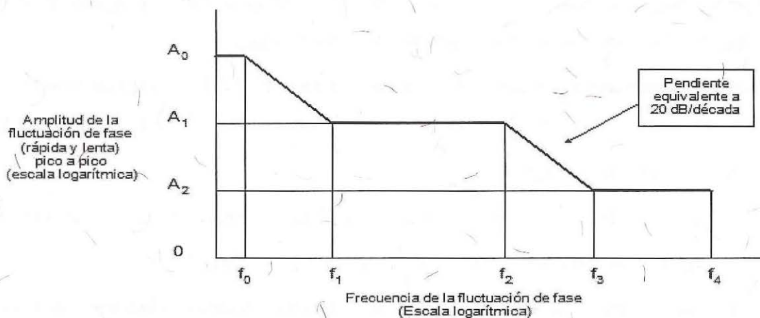
FIGURA B.2.- Límite inferior de la fluctuación de fase y fluctuación lenta de fase máxima
