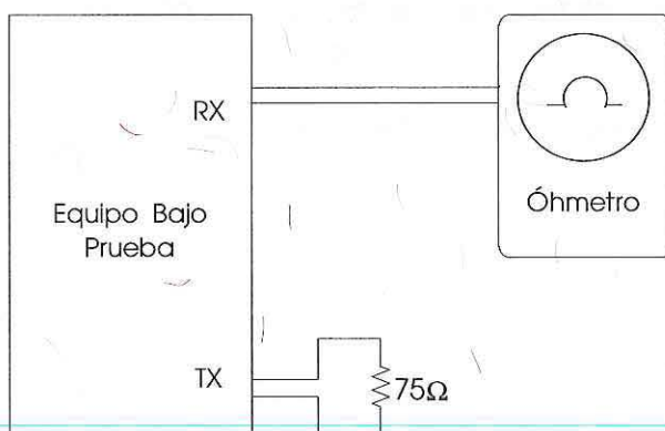
Figura 5.-Diagrama para la medición de la impedancia en el puerto de entrada
