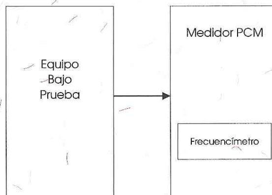
Figura 3.- Diagrama para la medición de la velocidad de transmisión
