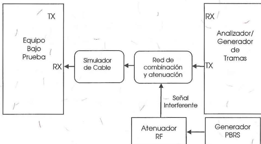
Figura 8. Diagrama para la verificar la tolerancia e inmunidad a una señal interferente
