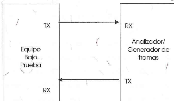
Figura 10. Diagrama para evaluar la estructura y señal de alineación de la trama básica
