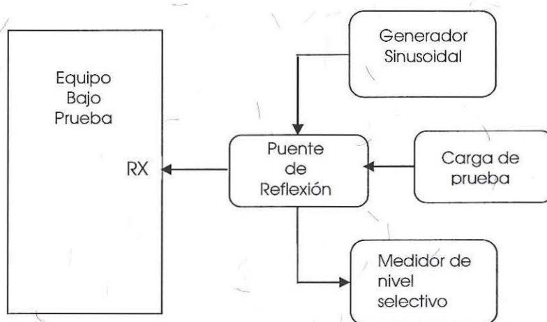
Figura 9. Diagrama para la medición de la pérdida de retorno en el puerto de entrada.
