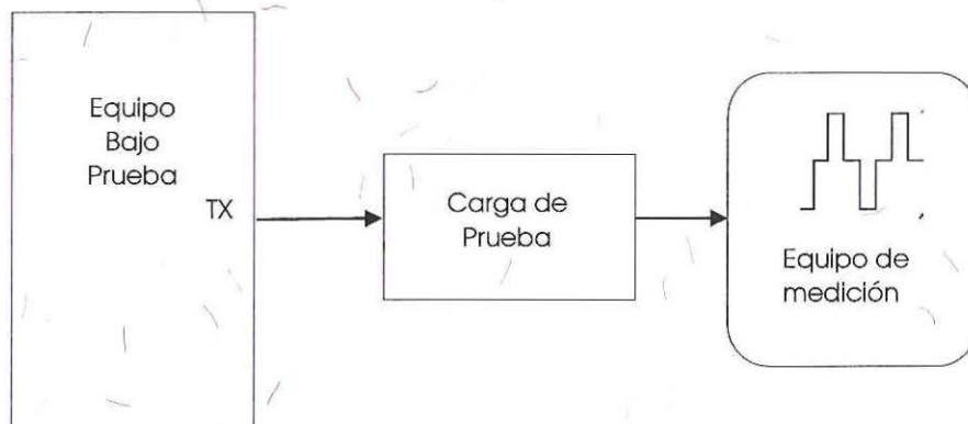
Figura 6.- Diagrama para la verificación de las características del pulso en el puerto de salida
